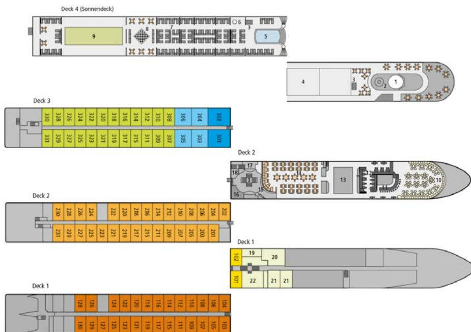
Beispiel Decksplan A-ROSA SILVA/FLORA
